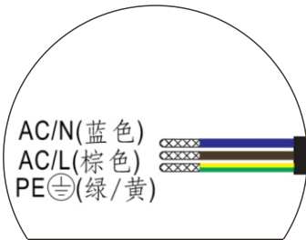
LED驱动电源线 颜色区分示意图
